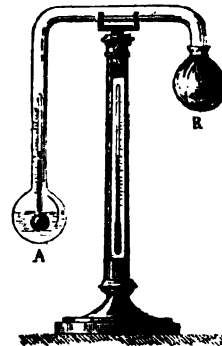
C. 1868. Hygrometr Daniellův.
